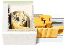
FR 59 in Einputzausführung
